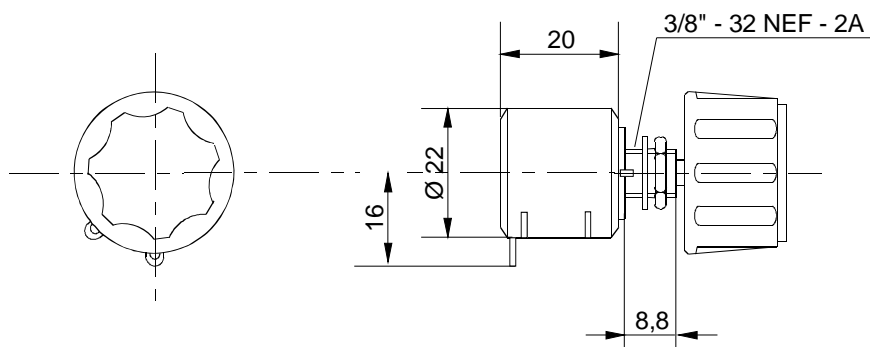
Abbildung 6: Potentiometer SW 02 - 10
