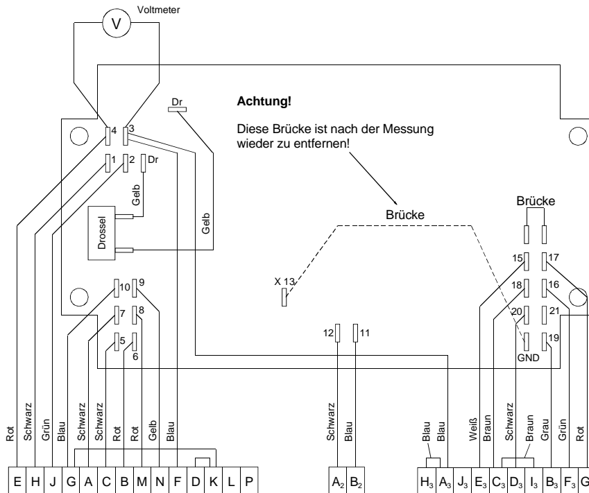
Abbildung 17: Interne Reglerverkabelung
