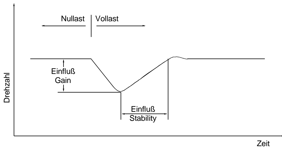
Abbildung 32: Einfluss der Dynamikparameter
