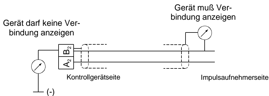
Abbildung 21: Beispiel Impulsnehmer Abschirmungsprüfung
