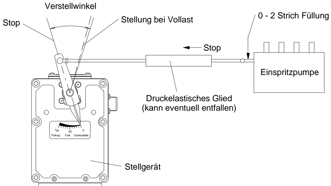
Abbildung 12: Gestänge für Dieselmotoren
