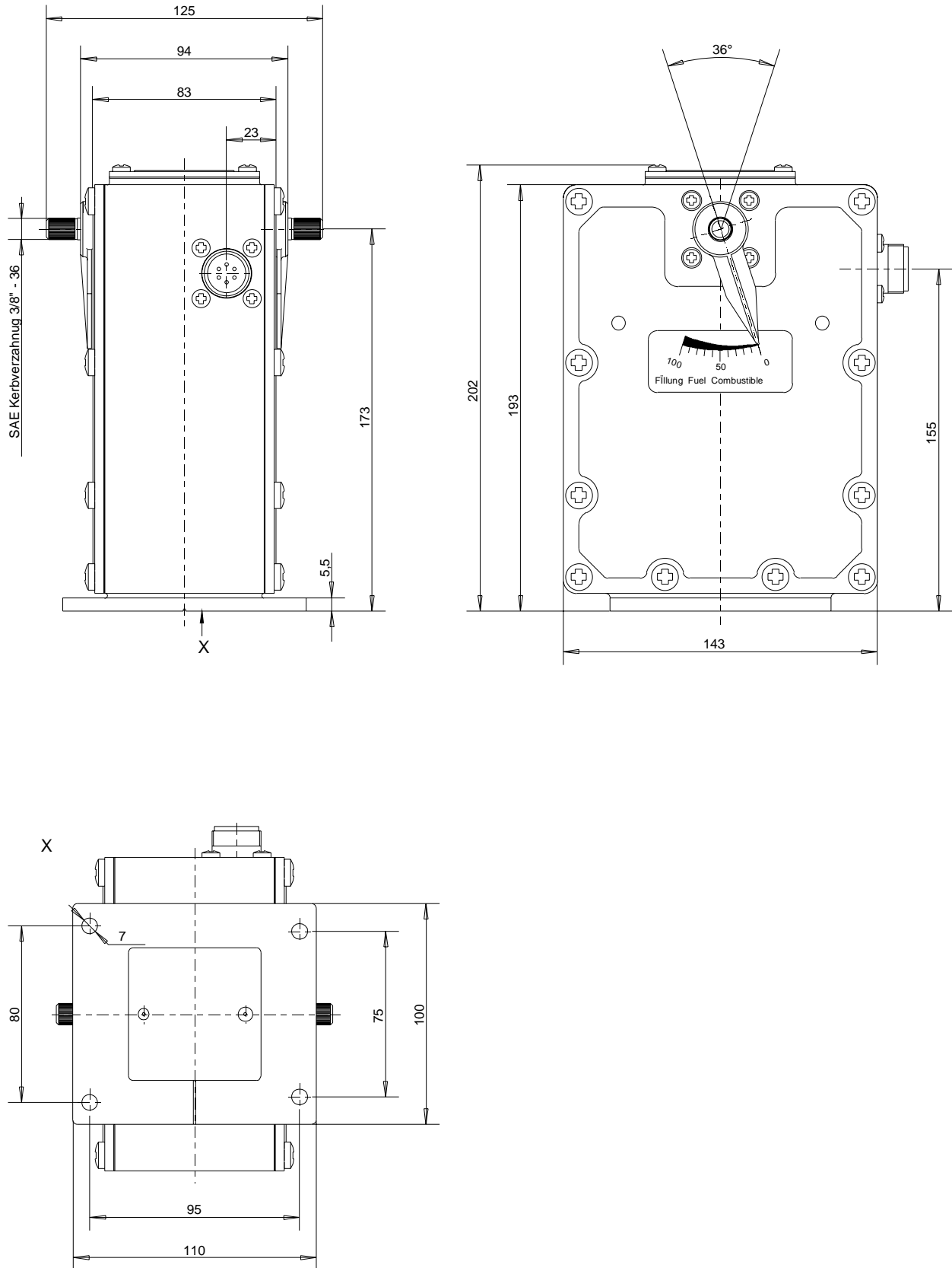
Abbildung 11: Stellgerät StG 10 - 01
