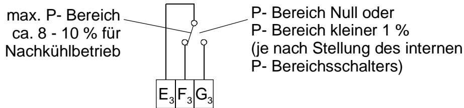
Abbildung 31: P- Bereichsummschaltung bei SB- Anlage
