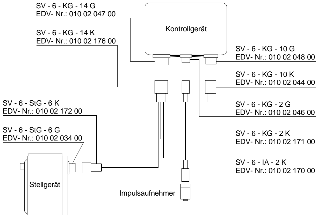
Abbildung 26: Steckerbezeichnungen
