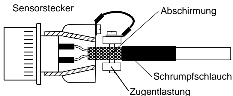
Abbildung 24: Beispiel einer Schirmbefestigung im Stecker
