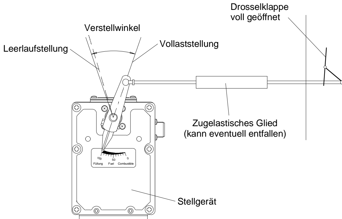
Abbildung 13: Gestänge für Gasmotoren
