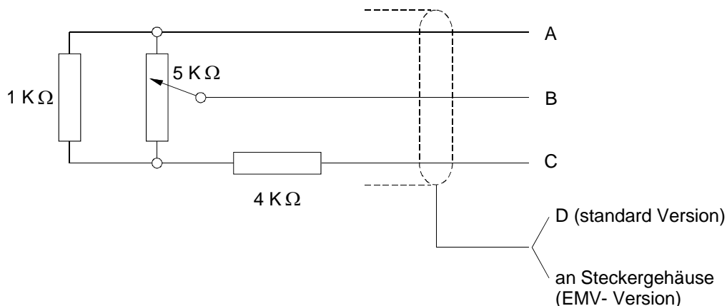
Abbildung 7: Anschluss der Bereichsbegrenzungswiderstände
