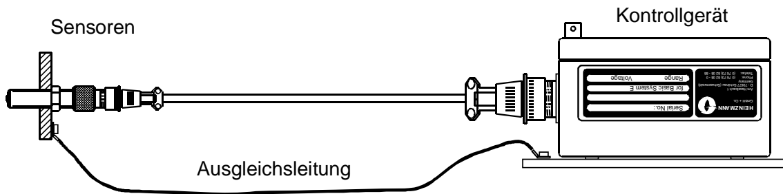
Abbildung 22: Anschluss einer Ausgleichsleitung
