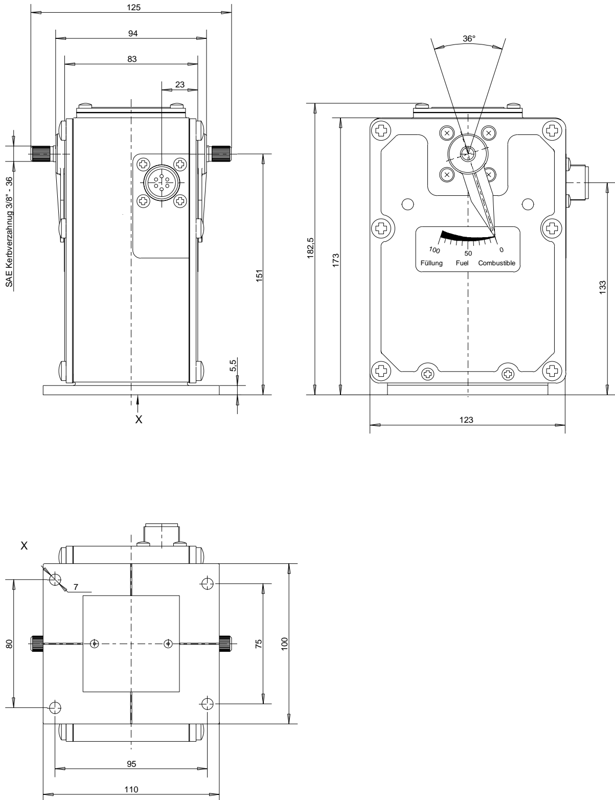
Abbildung 10: Stellgeräte StG 6 - 01 und StG 6 - 02 - V
