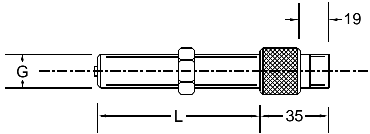
Abbildung 4: Impulsaufnehmer
