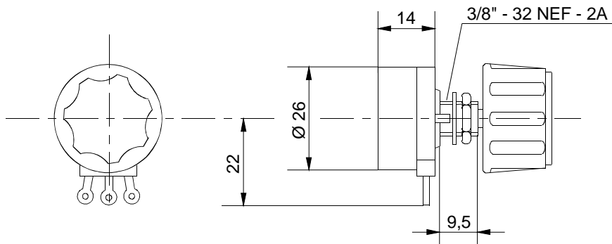
Abbildung 5: Potentiometer SW 01 - 1
