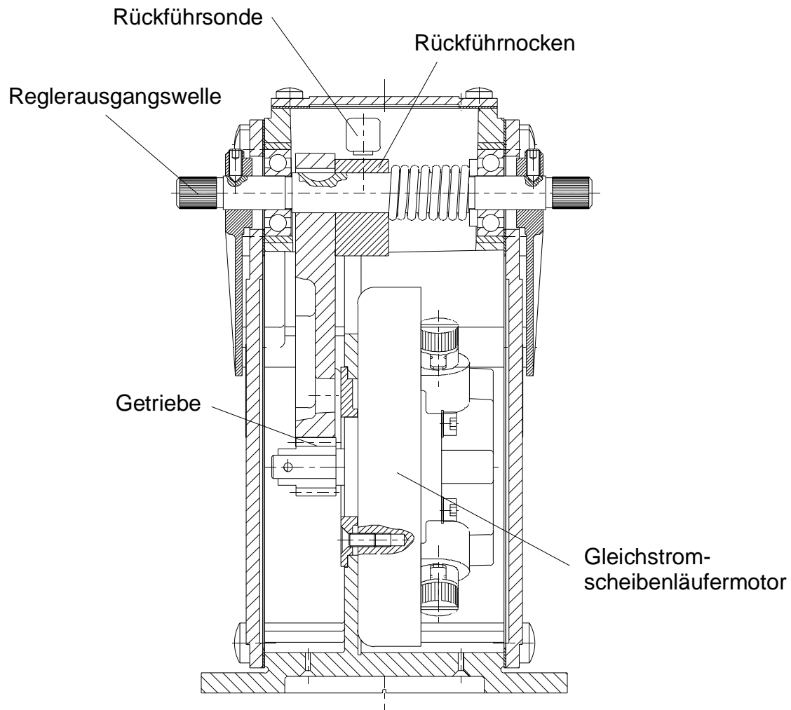
Abbildung 9: Schnittzeichnung des Stellgerätes
