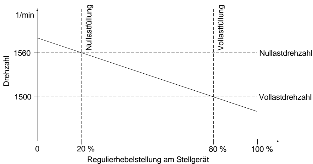
Abbildung 29: P- Bereich
