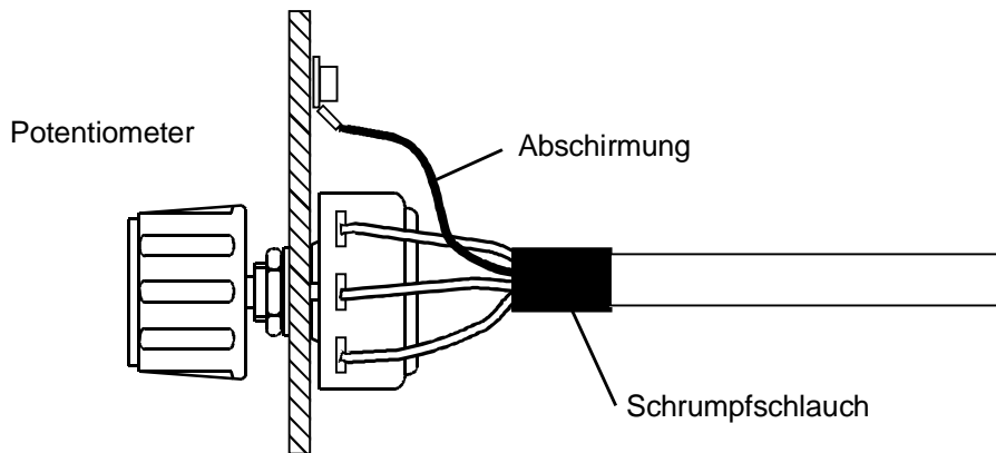
Abbildung 23: Beispiel einer Schirmbefestigung ohne Stecker
