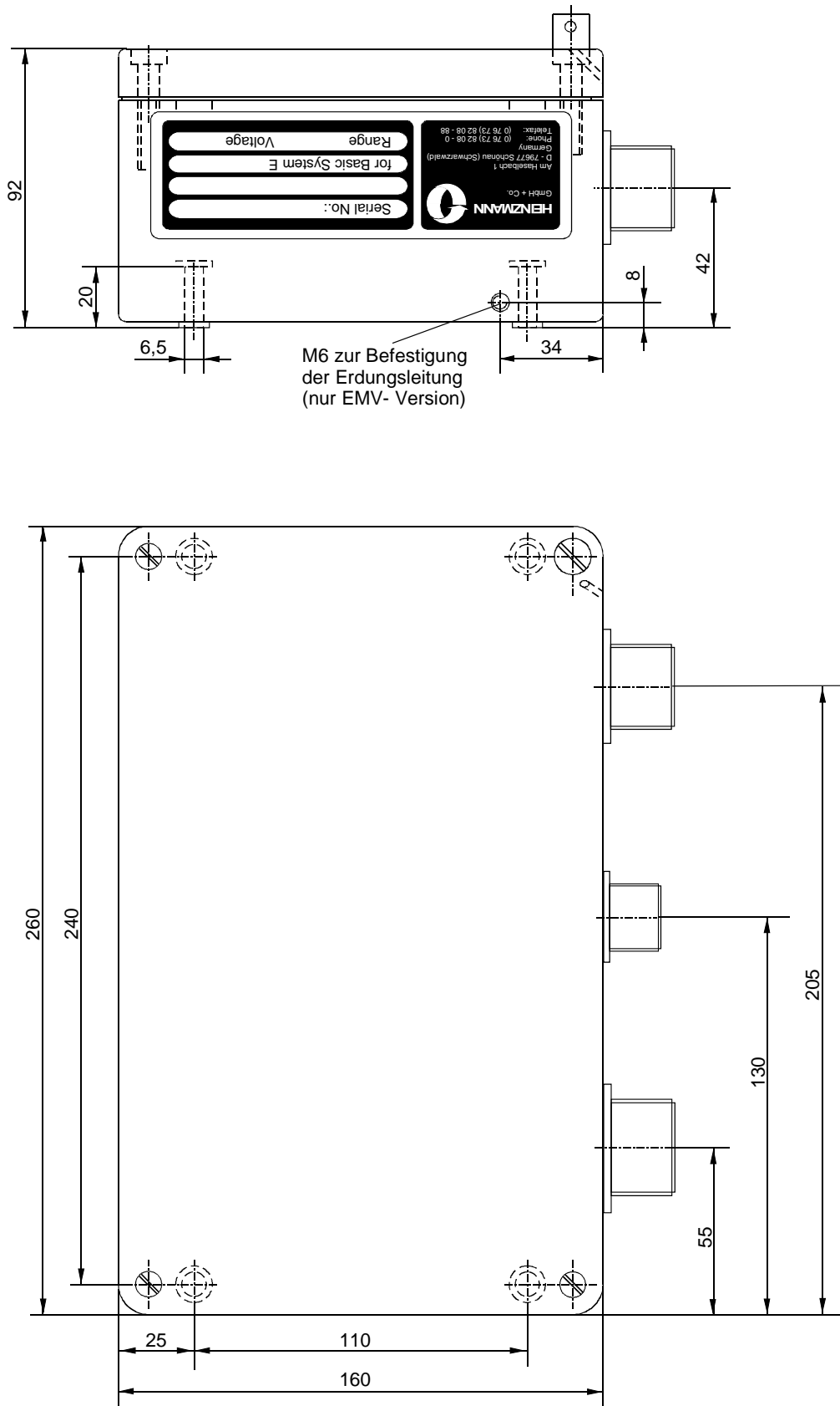
Abbildung 8: Gehäuse des KG 6 - 04 bis KG 10 - 04
