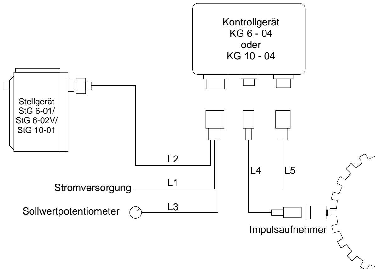
Abbildung 25: Kabellängen für E 6 bis E 10
