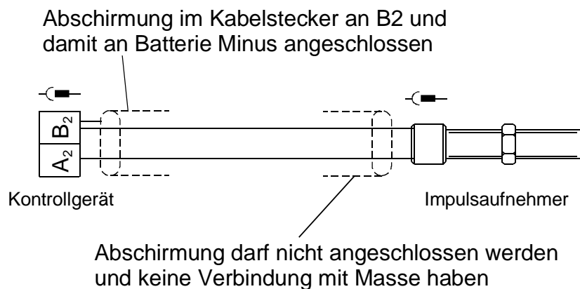
Abbildung 18: Abschirmung Impulsaufnehmer ohne EMV
