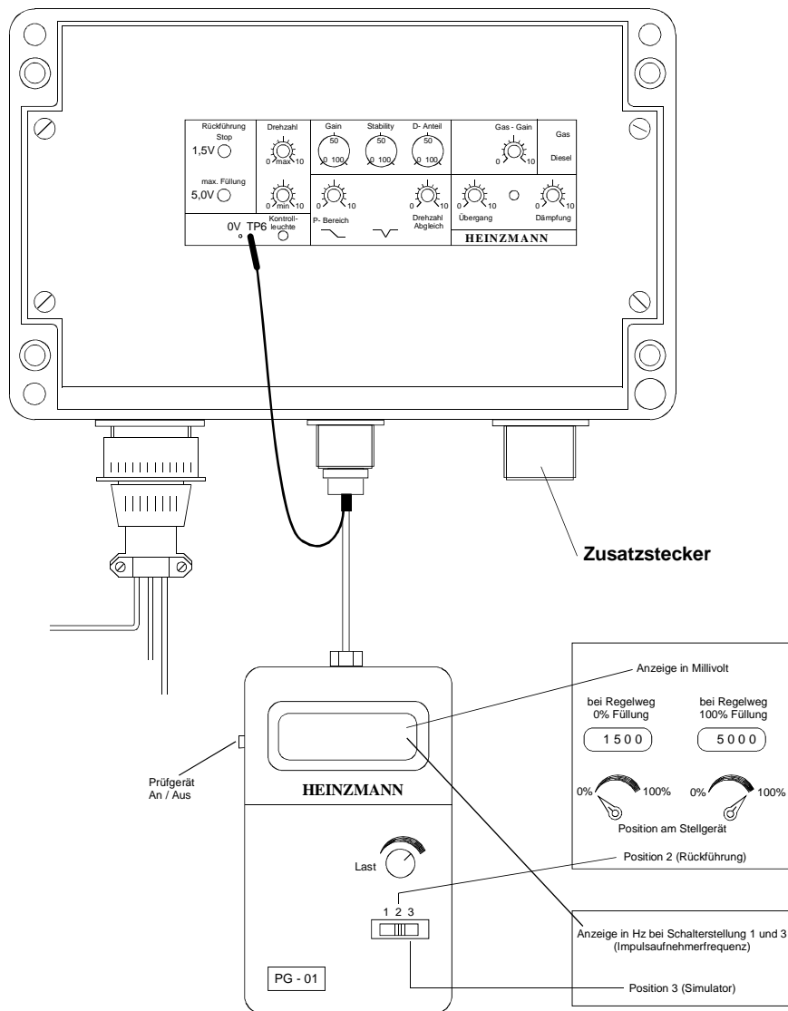
Abbildung 28: Anschluss des Prüfgerätes PG 01 an das Kontrollgerät
