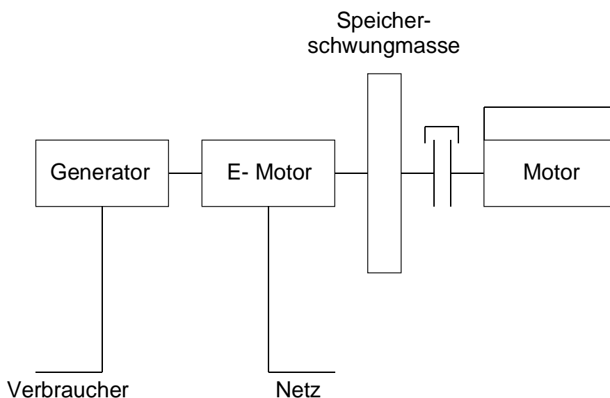
Abbildung 30: Sofortbereitschaftsanlage
